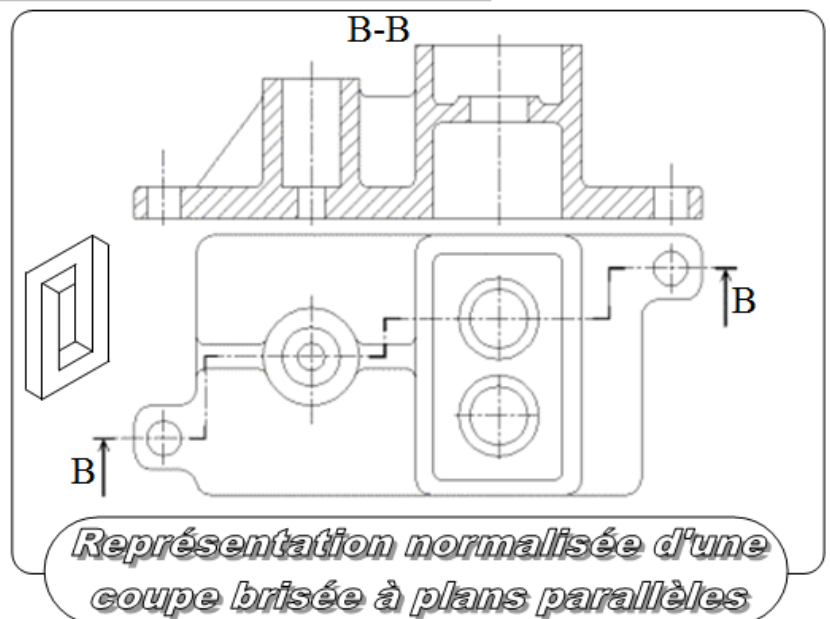
Coupe brisée à plans parallèles
